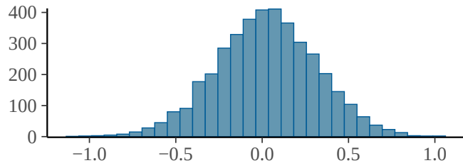
b_B_AUC.bl
