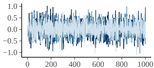
b_B_AUC.bl
